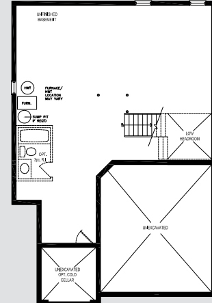
BASEMENT PLAN EL 'A'
